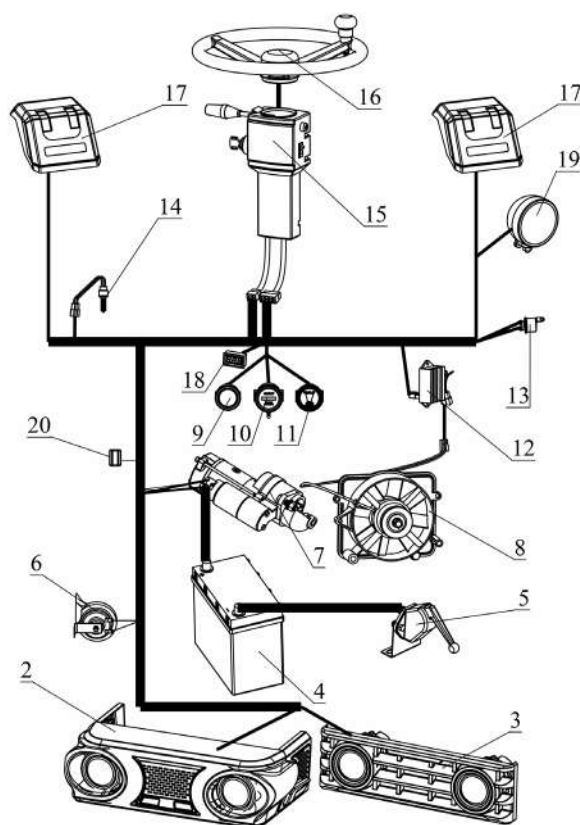
Рис. 23. Схема электрооборудования тракторов Кентавр
