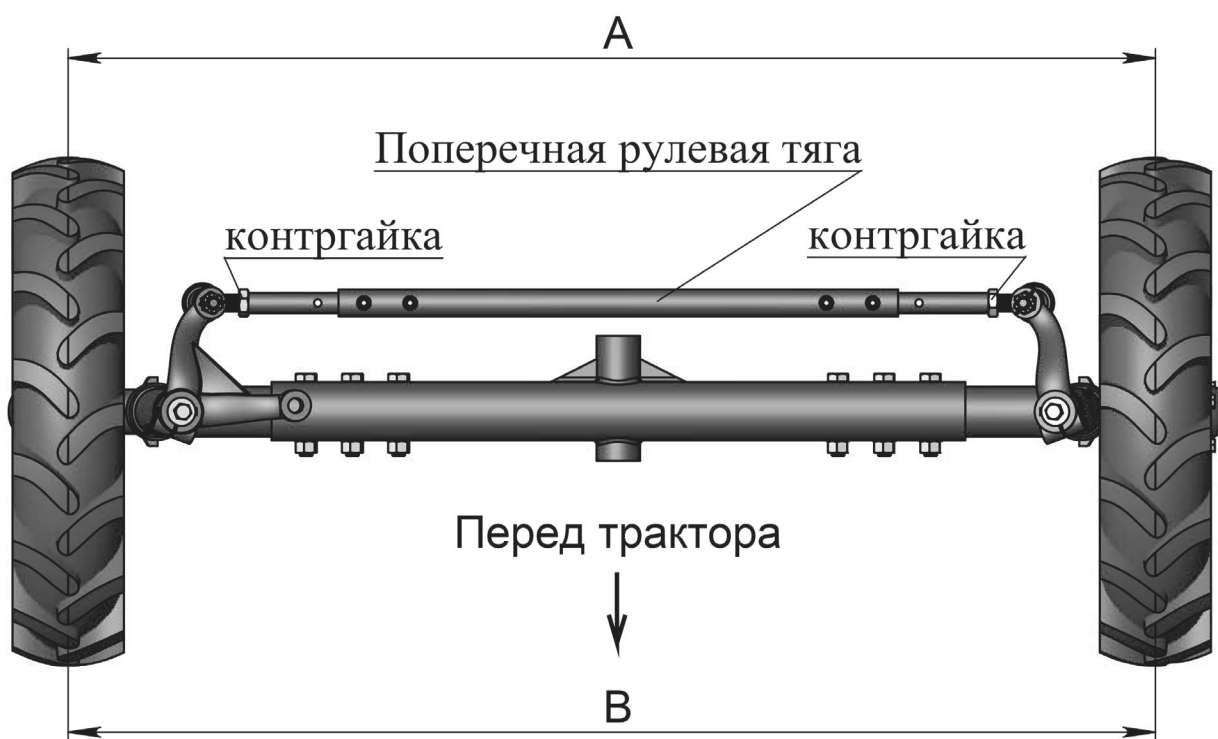
Рис. 14. Регулировка схождения передних колес
