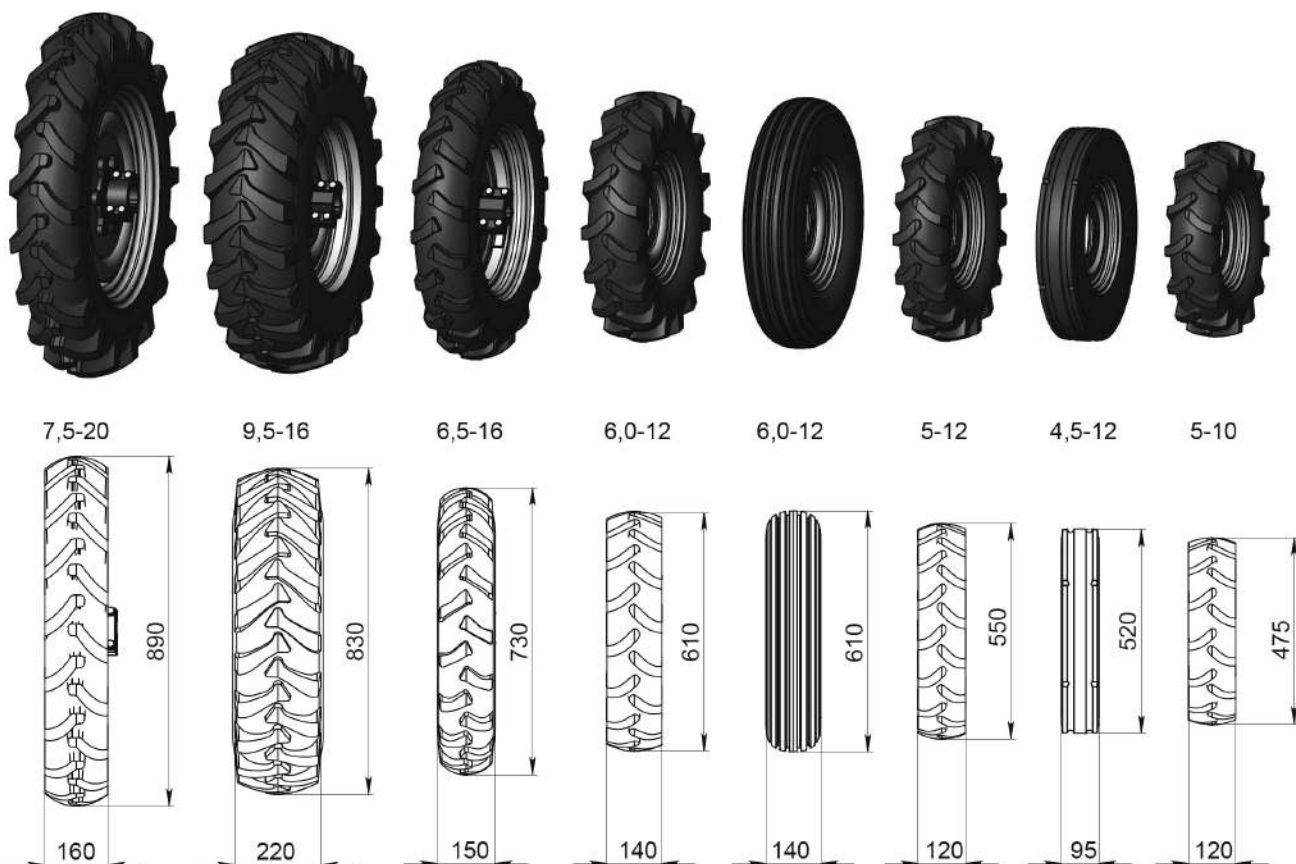
Рис. 18. Размеры колес
